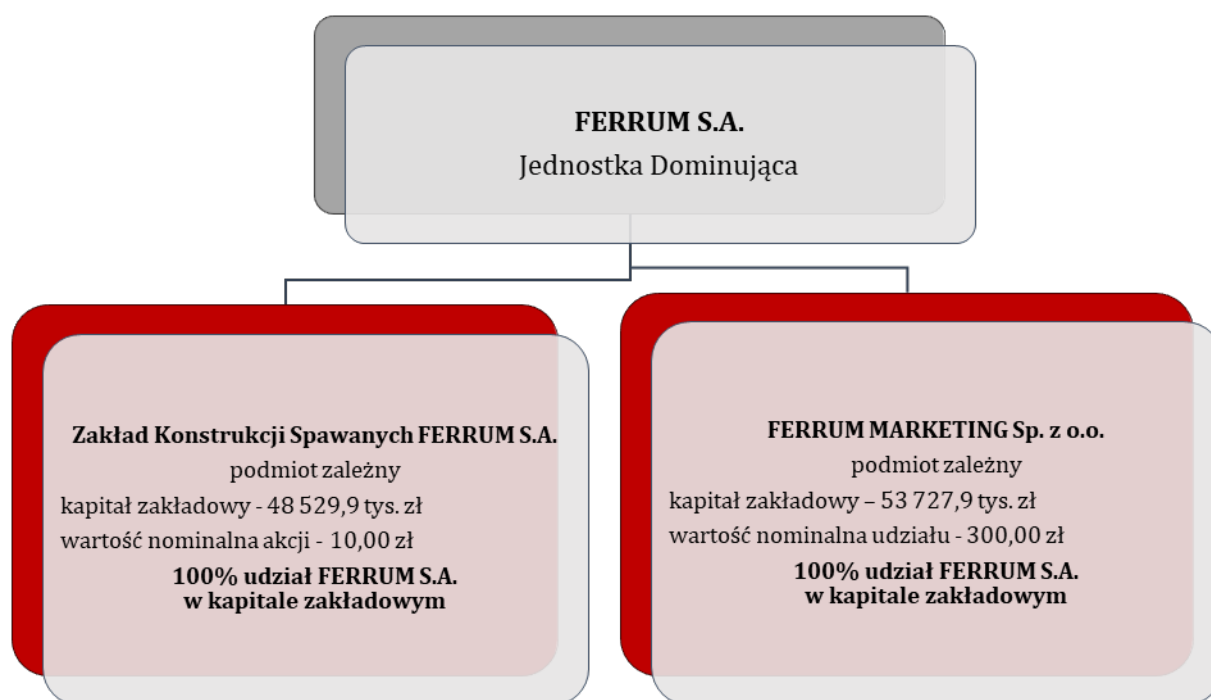
Rys. 3. Skład Grupy Kapitałowej FERRUM na dzień 31 grudnia 2020 r.
