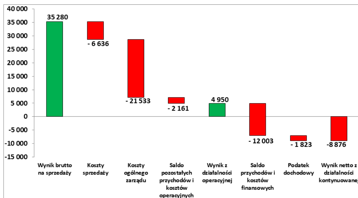
Rys. 1. Składowe skonsolidowanego wyniku netto za 2020 r. (w tys. zł)
