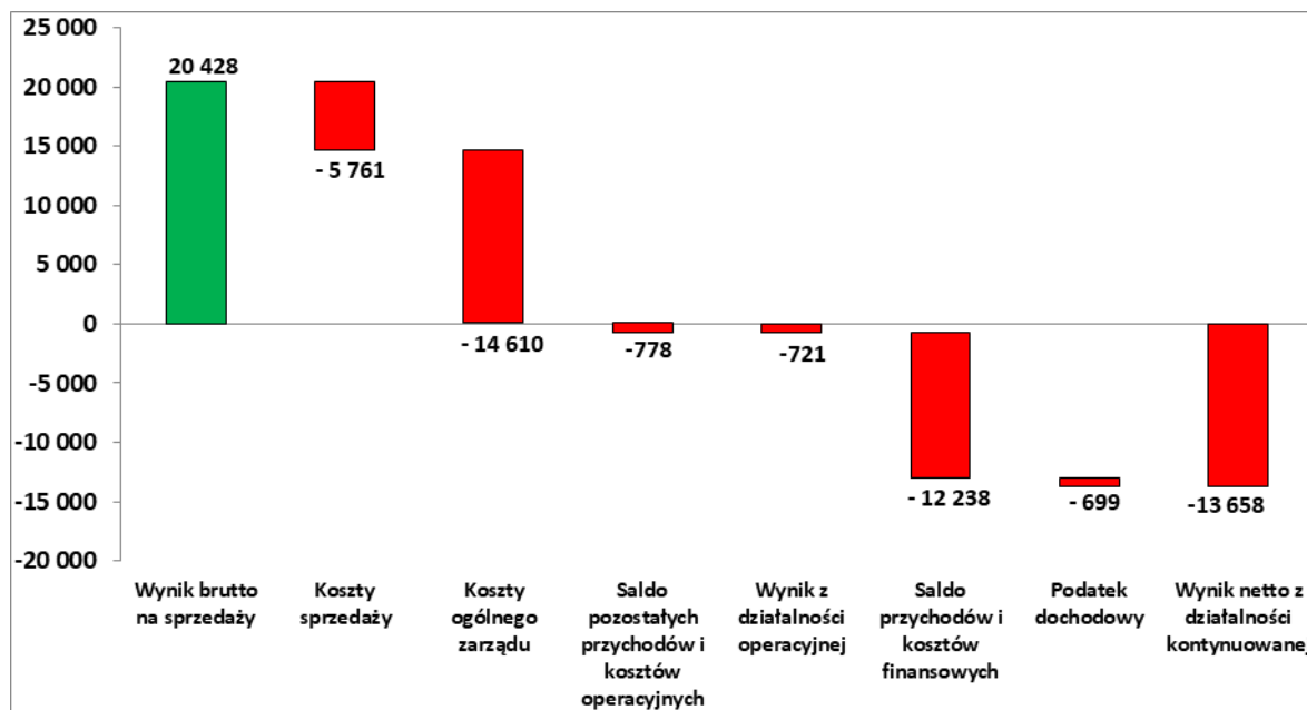
Rys. 2. Składowe jednostkowego wyniku netto za 2020 r. (w tys. zł)
